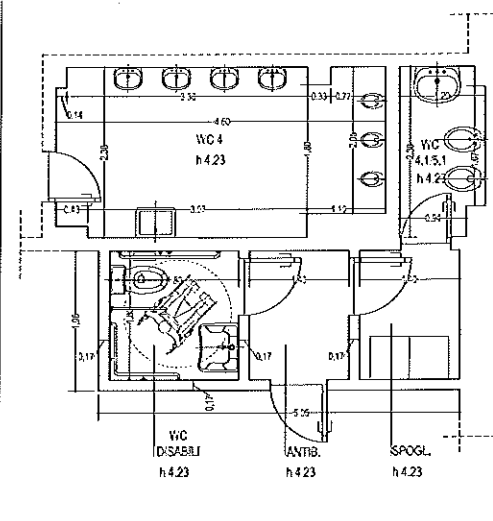
PARTICOLARE 4 SCALA 1:50
