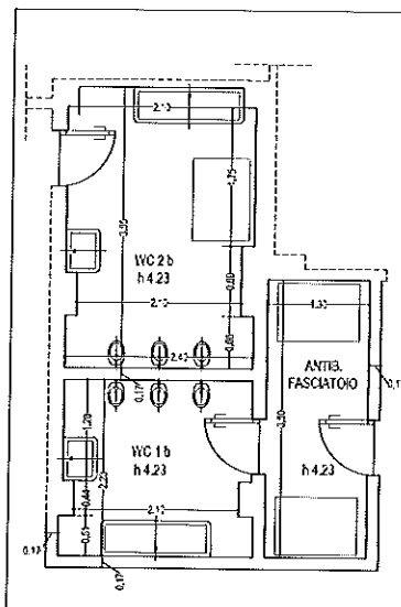
PARTICOLARE 7 SCALA 1:50
