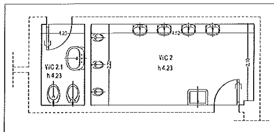
PARTICOLARE 2 SCALA 1:50
