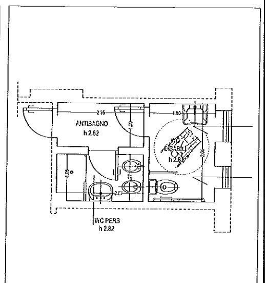
PARTICOLARE 8 SCALA 1:50
