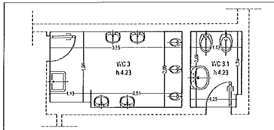
PARTICOLARE 3 SCALA 1:50
