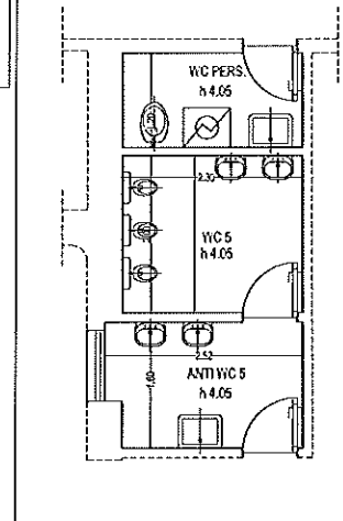
PARTICOLARE 5 SCALA 1:50
